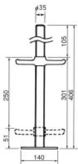
大引受ジャッキ A-752H 5.3kg
