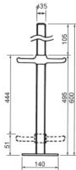
ピボットジャッキ PB-14J 3.7kg
